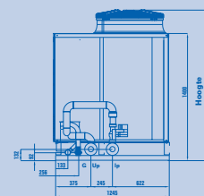
Vooraanzicht
