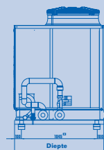
Zijaanzicht rechts L2 cascade
