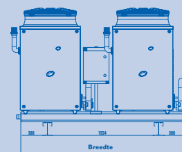
Vooraanzicht L2 cascade
