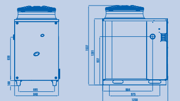
Vooraanzicht
